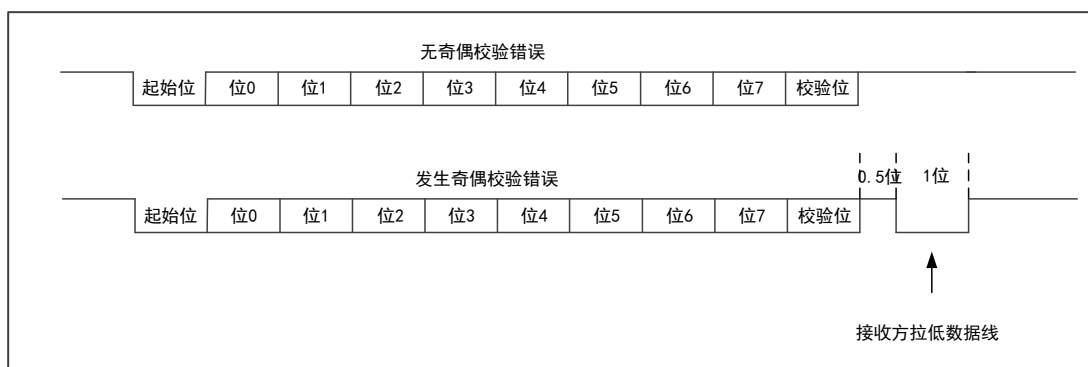
图 91 ISO7816-3 标准协议
