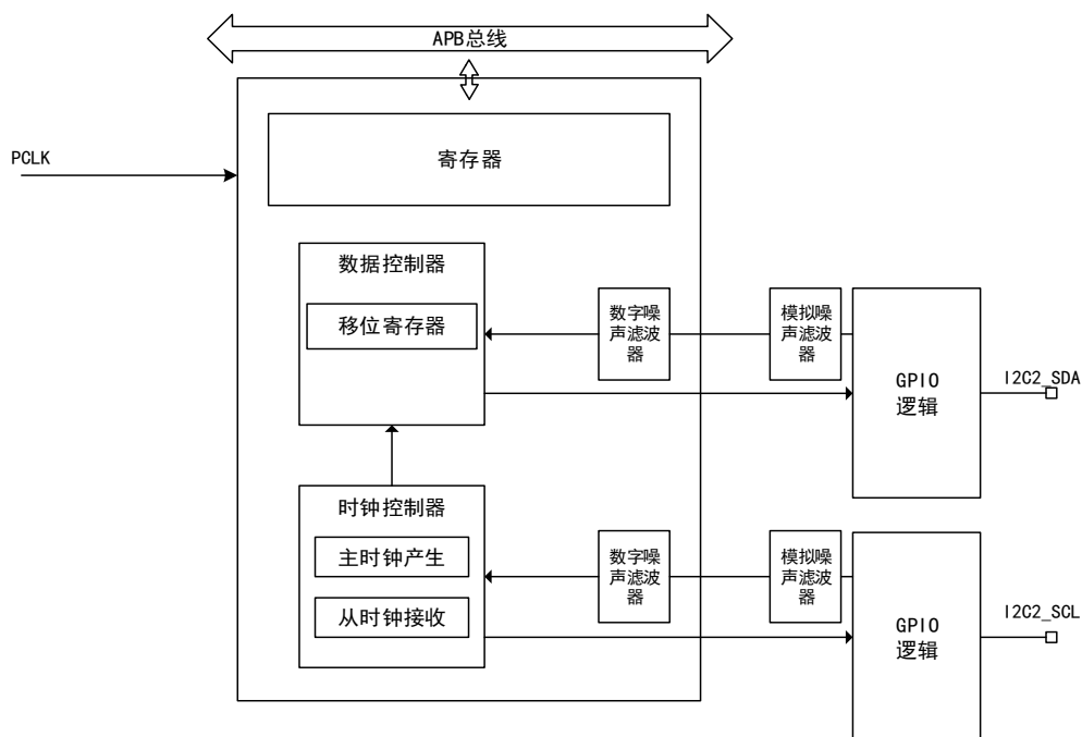
图 96 I2C2 功能结构图
