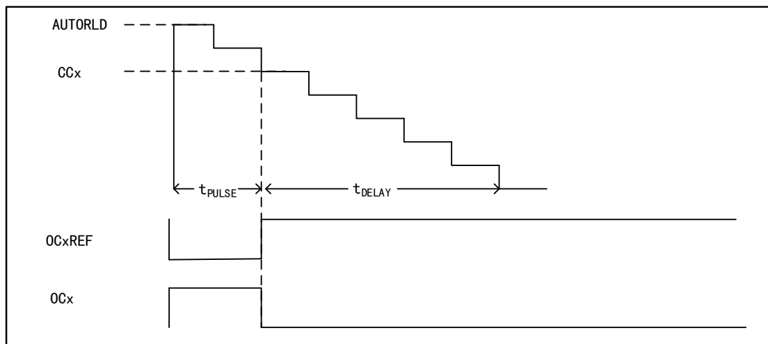
图 52 单脉冲模式下的时序图
