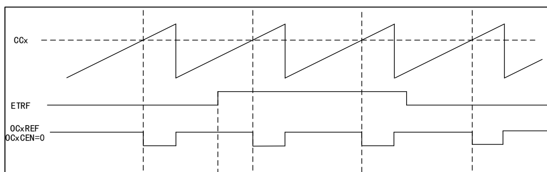
图 76 OCxREF 时序图
