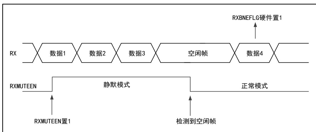
图 83 空闲总线退出静默模式
