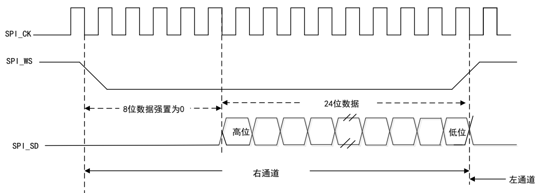
图 112 LSB 对齐标准波形（24 位数据）
