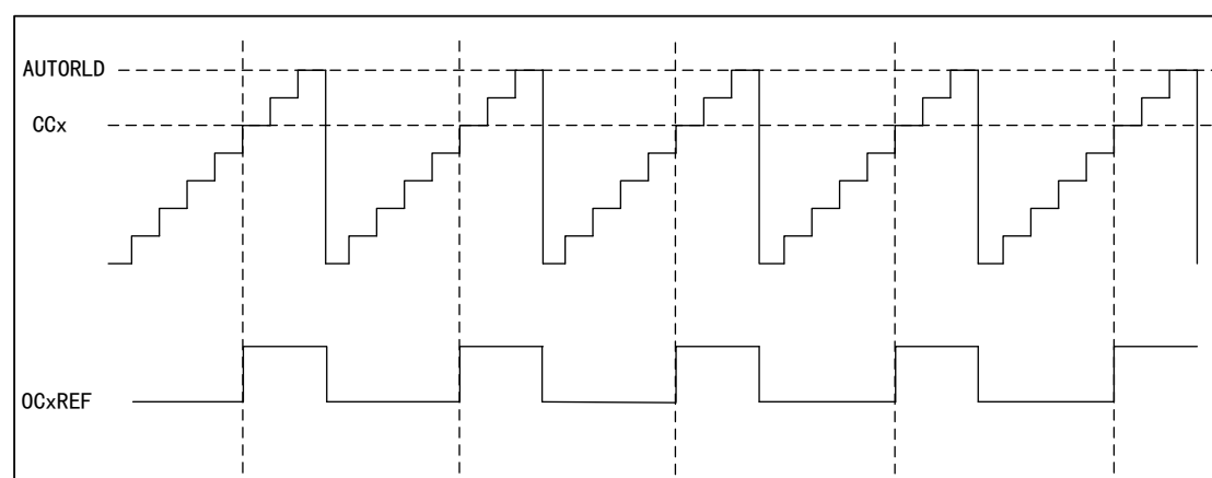
图 65 PWM2 向上计数模式的时序图
