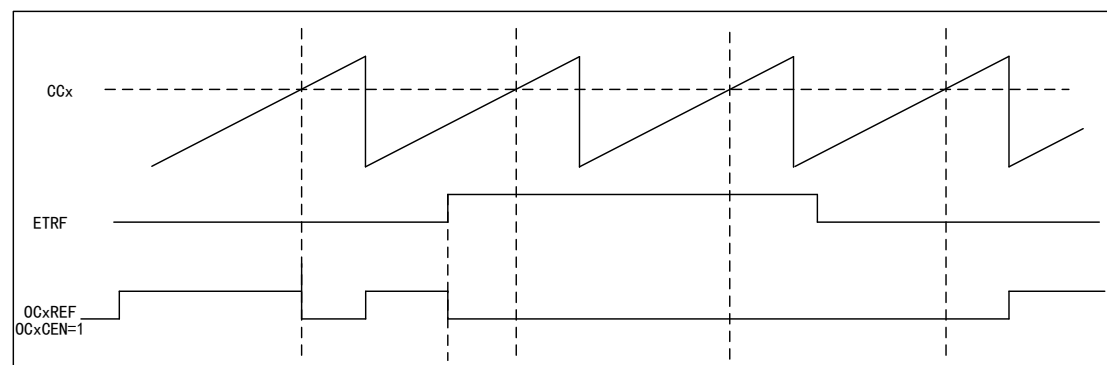
图 77 OCxREF 时序图
