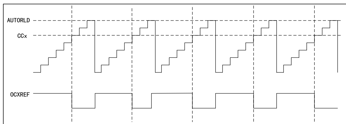
图 49 PWM1 向上计数模式的时序图
