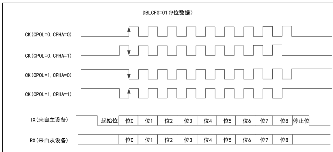
图 88 USART 同步传输时序图 (DBLCFG=01)
