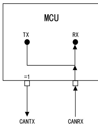
图 118 CAN 工作在静默模式
