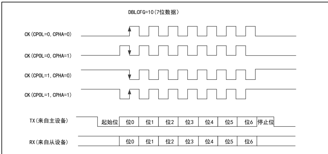
图 86 USART 同步传输时序图 (DBLCFG=10)
