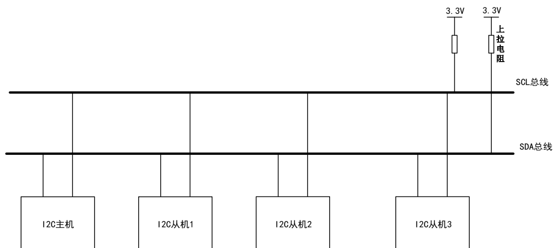
图 97 常见 I2C 通信连接图
