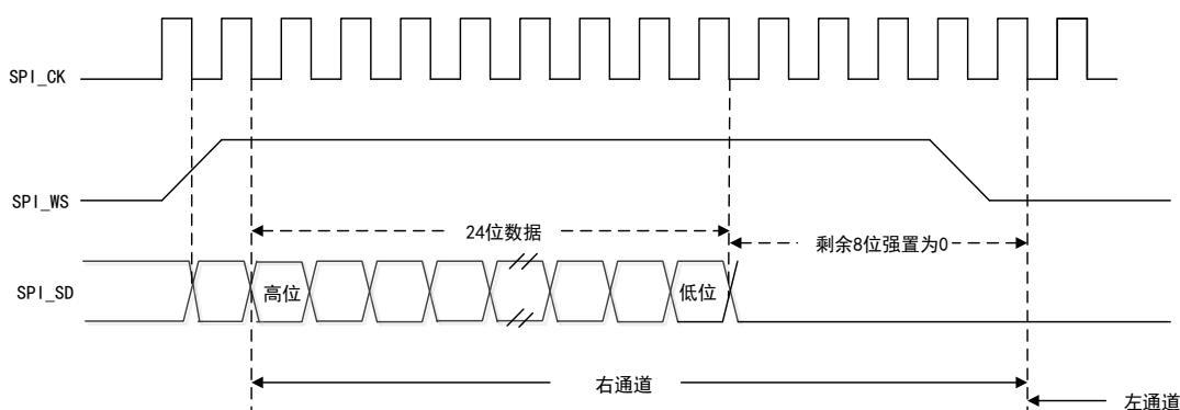
图 106 I2S 飞利浦协议波形（24 位）
