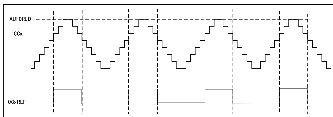
图 67 PWM2 中央对齐模式的时序图
