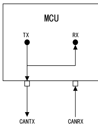
图 119 CAN 工作在环回模式
