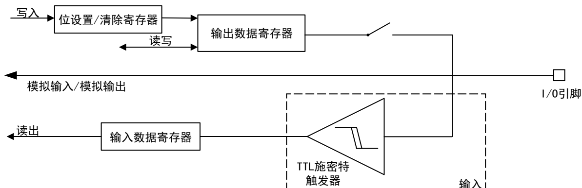
图 21 模拟功能 I/O 结构
