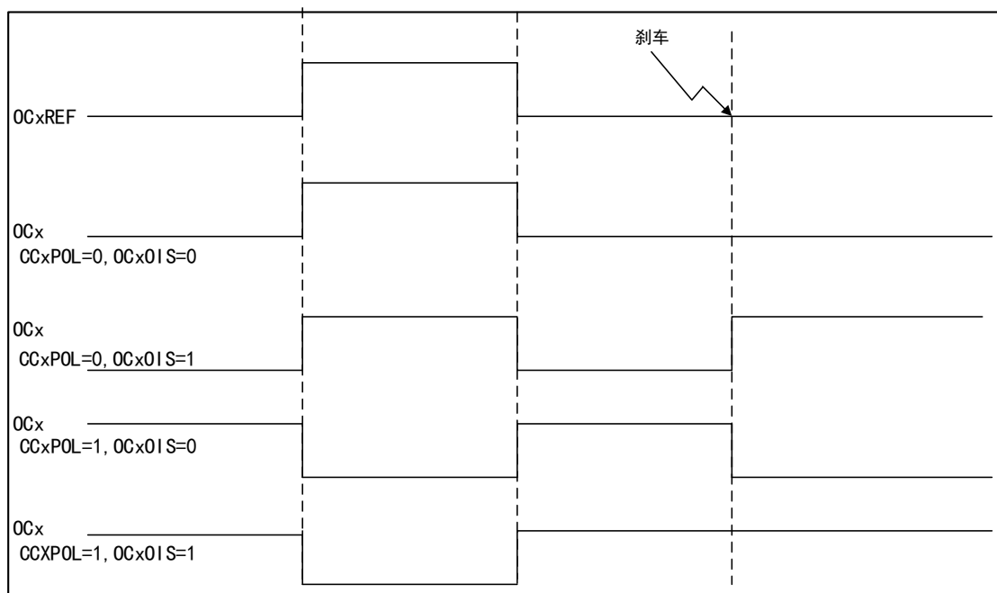
图 54 发生刹车事件的时序图
