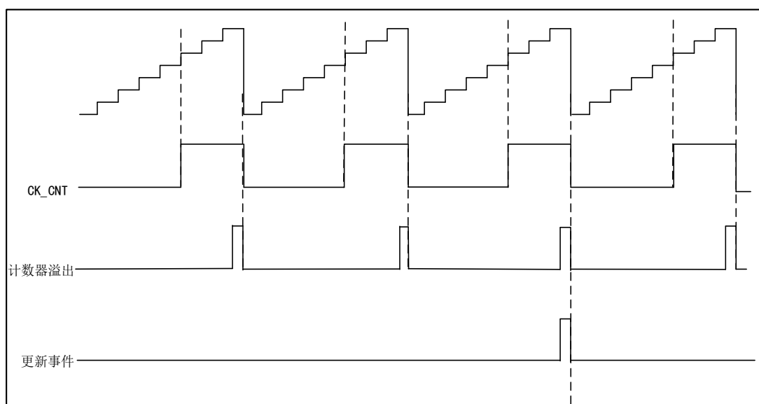
图 61 向上计数模式下，设置 REPCNT=2 的时序图
