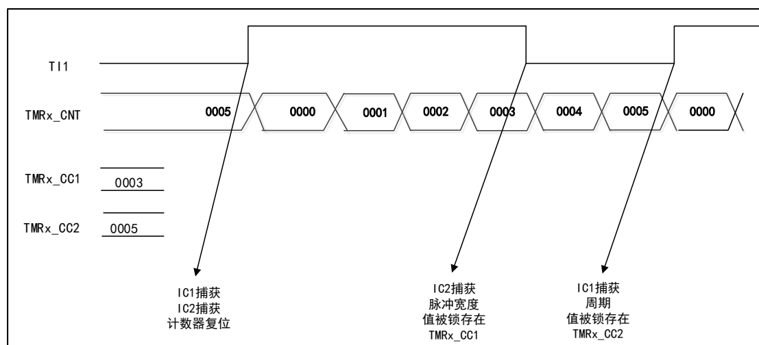
图 51 PWM 输入模式时序图
