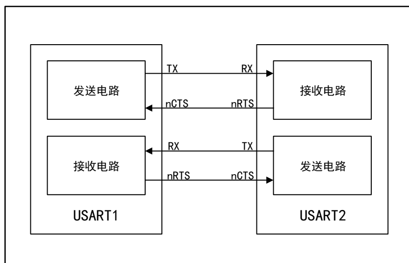
图 93 两个 USART 之间的硬件流控制
