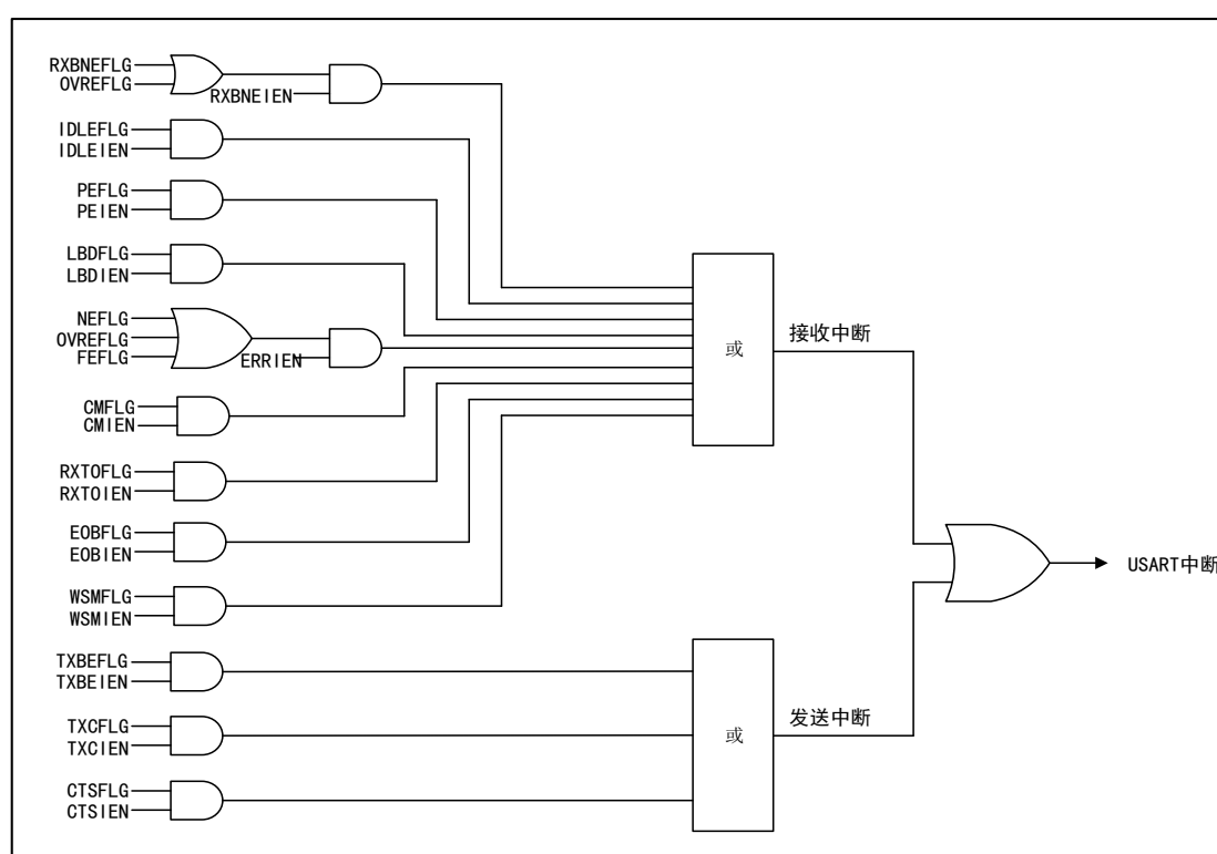
图 94 USART 中断映射
