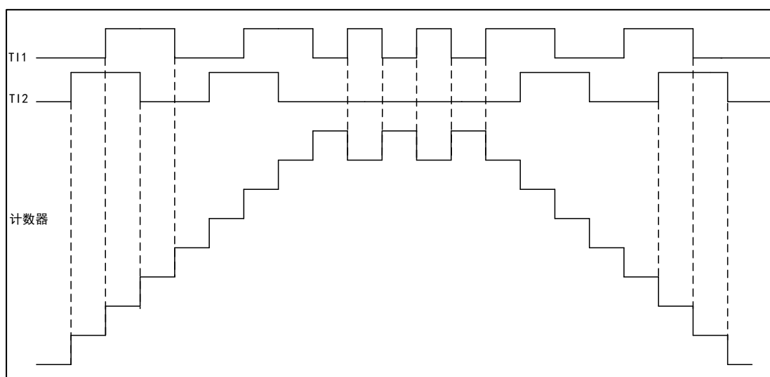
图 73 编码器模式下的计数器操作实例
