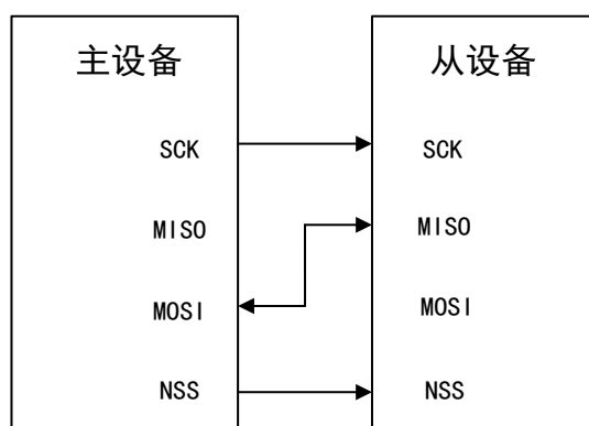
图 102 半双工模式连接
