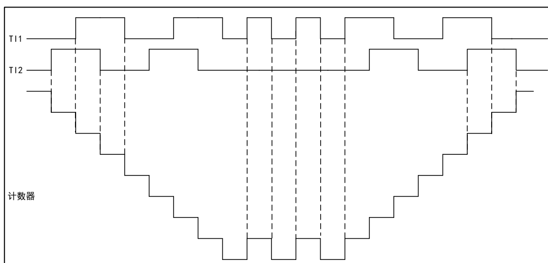
图 74 IC1FP1 反相的编码器接口模式实例
