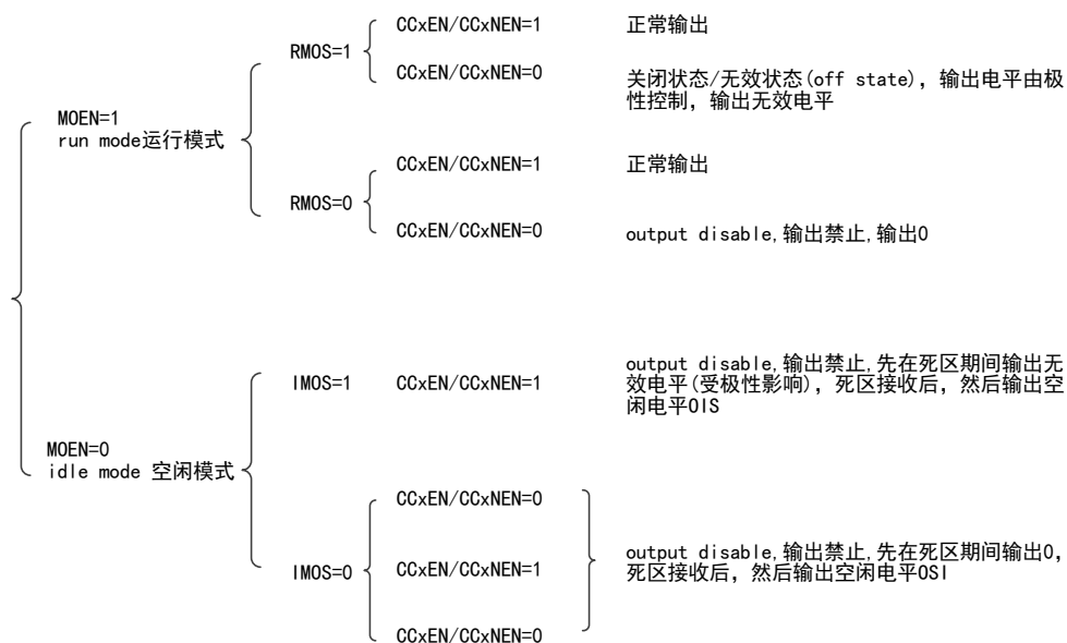
图 53 影响输出波形的寄存器结构关系
