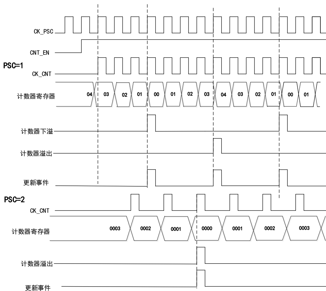
图 60 中央对齐模式下，分频因子为 1 或 2 的时序图
