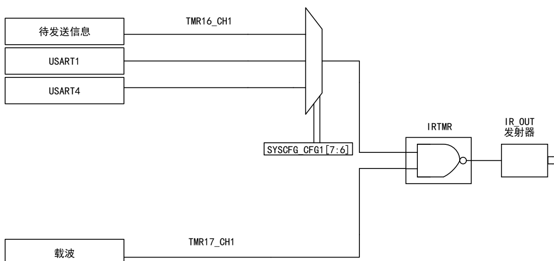
图 78 IRTMR 结构框图
