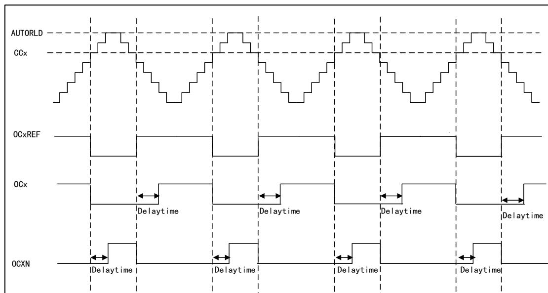
图 55 带死区插入的互补输出
