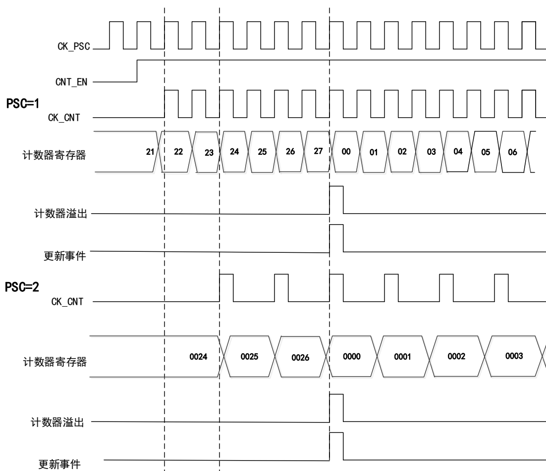
图 58 向上计数模式下，分频因子为 1 或 2 的时序图
