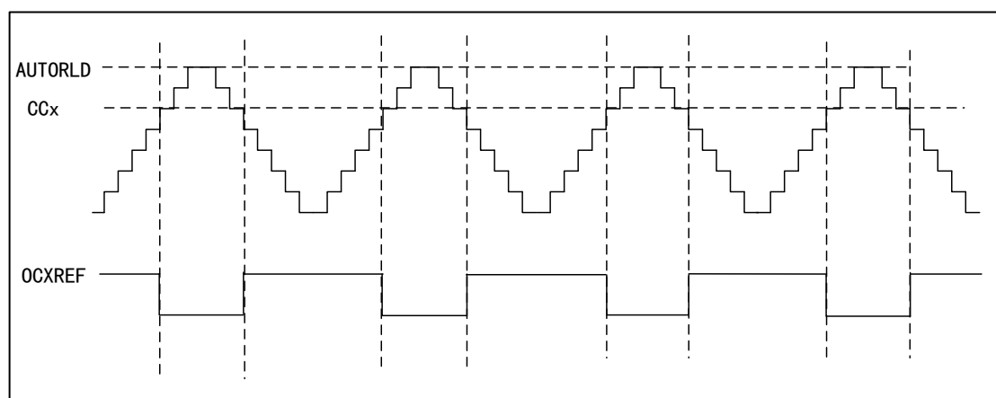
图 64 PWM1 中央对齐模式的时序图
