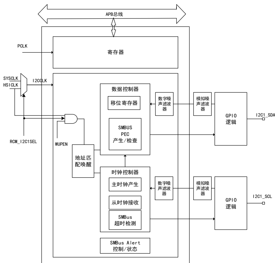
图 95 I2C1 功能结构图
