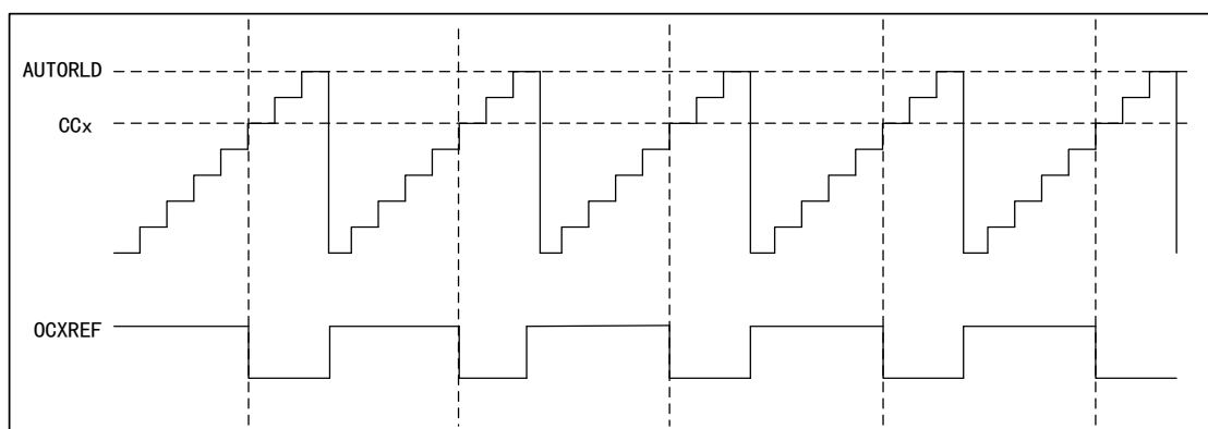
图 43 PWM1 向上计数模式的时序图
