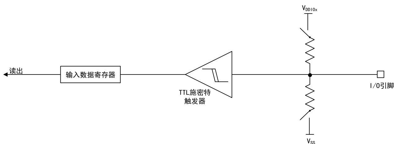
图 18 输入模式 I/O 结构
