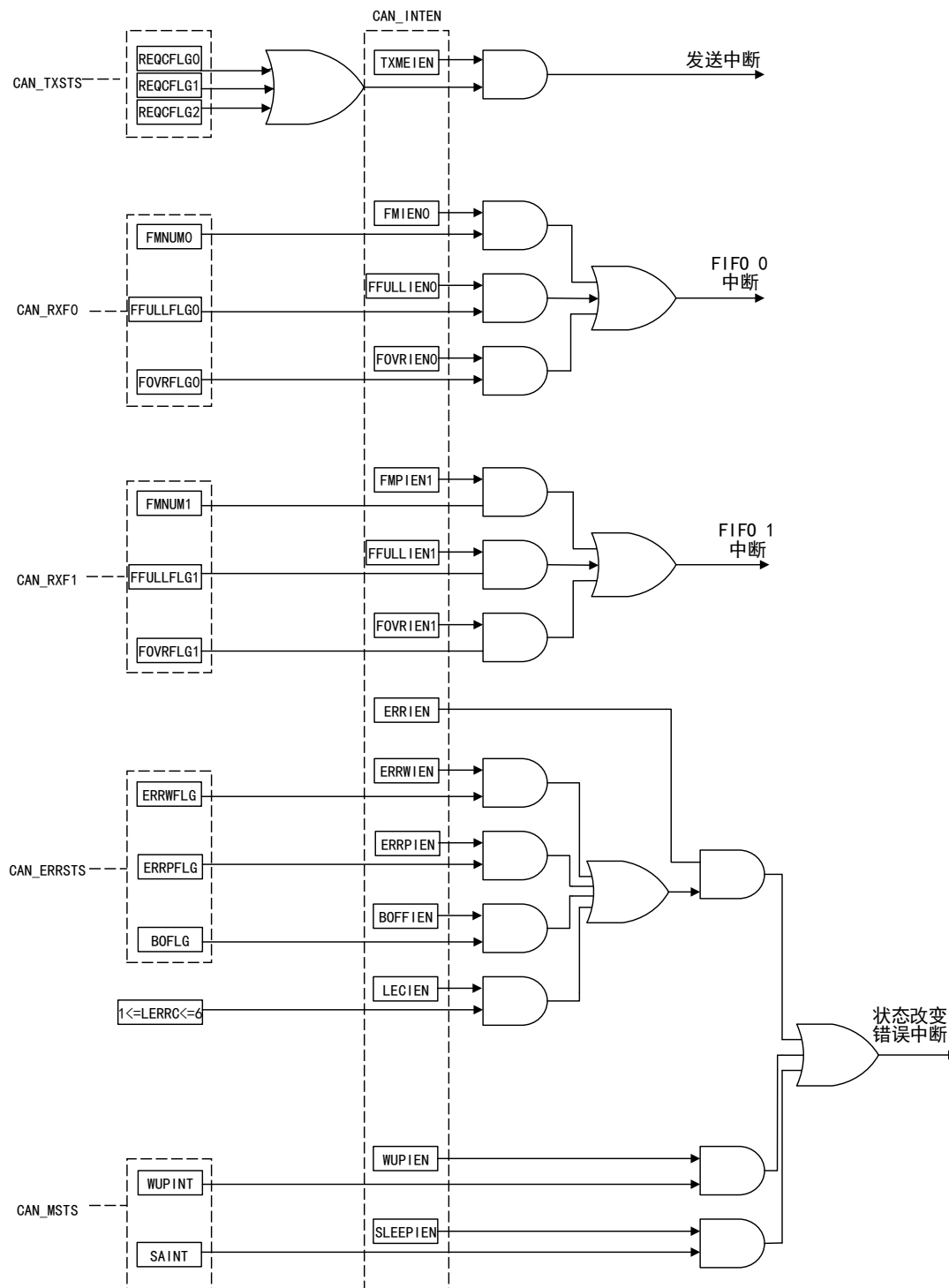
图 124 事件标志和中断产生
