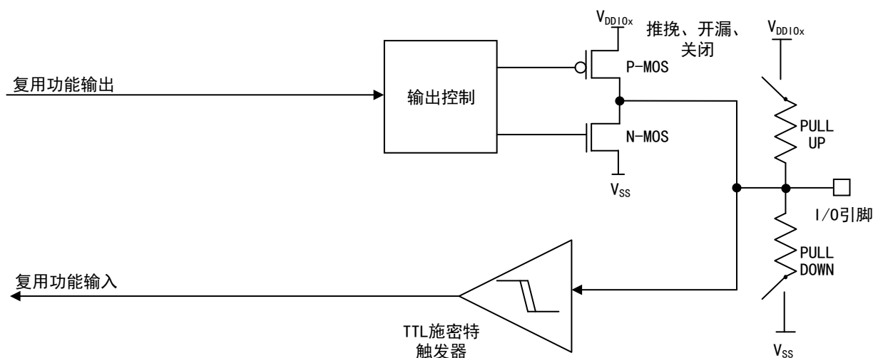
图 20 复用模式 I/O 结构
