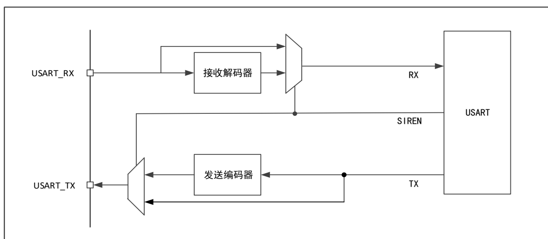
图 92 IrDA 模式框图
