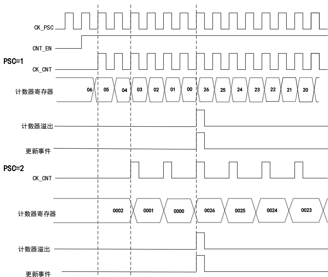
图 59 向下计数模式下，分频因子为 1 或 2 的时序图
