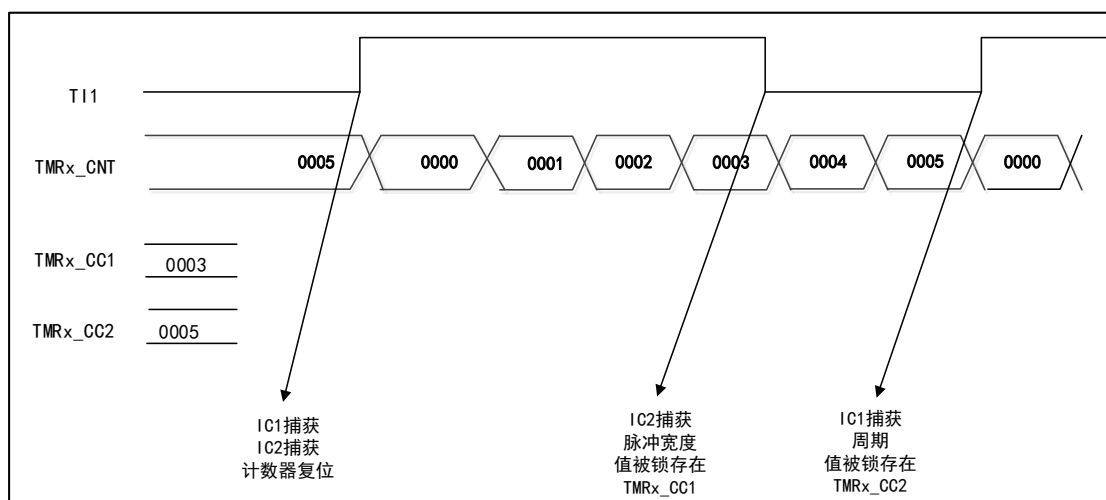
图 68 PWM 输入模式时序图
