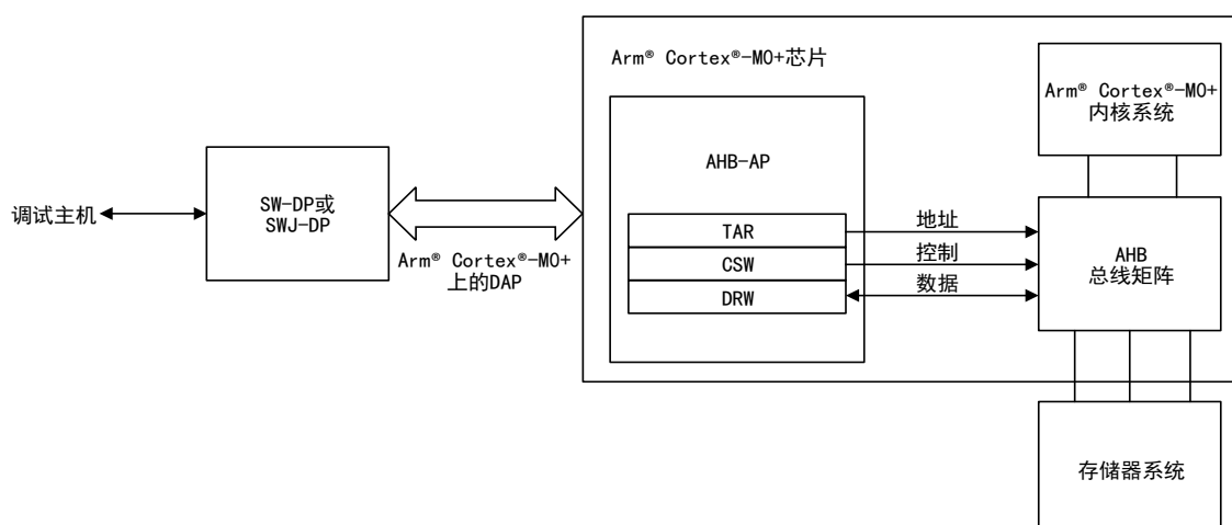
图 16 APM32A0xx 级别和 Arm® Cortex®-M0+级别的调试框图
