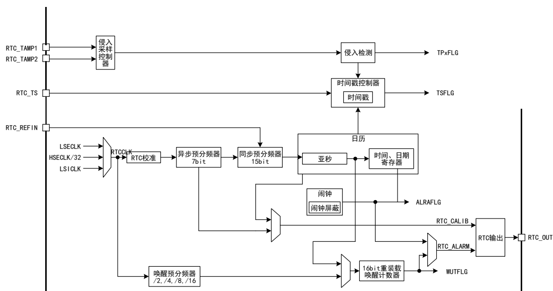
图 82 RTC 结构框图
