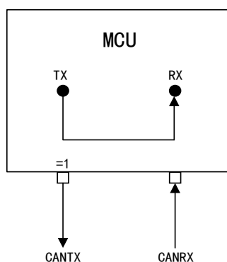
图 120 CAN 工作在静默环回模式
