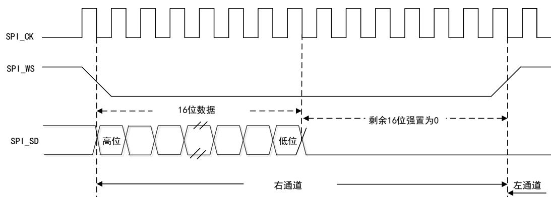
图 110 MSB 对齐标准波形（16 位扩展至 32 位）
