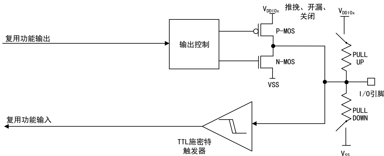
图 22 复用模式下的 I/O 结构
