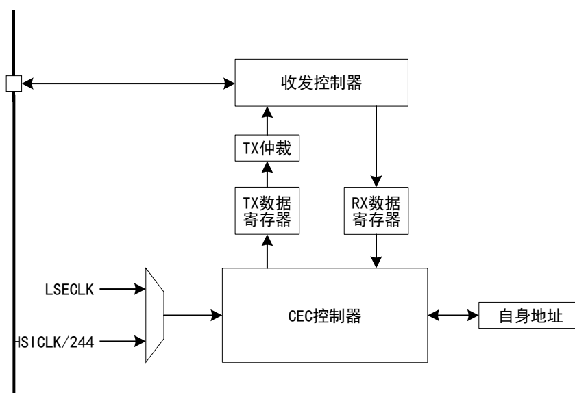
图 125 CEC 结构框图
