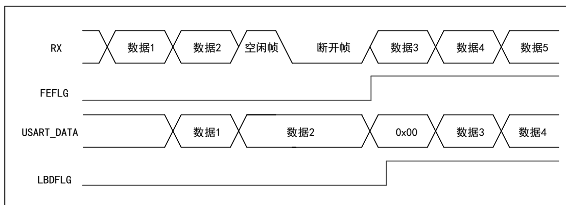
图 89 空闲状态检测断开帧
