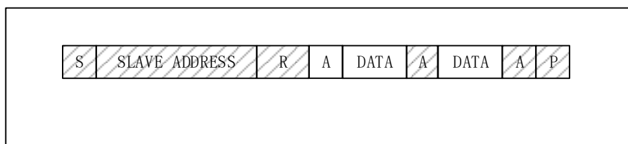
图 99 主机由从机读取数据
