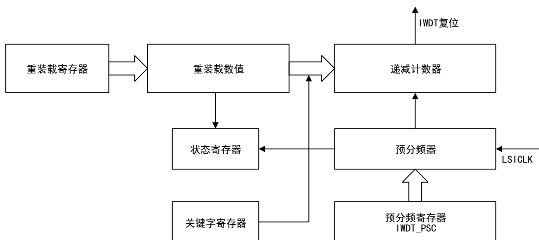
图 79 独立看门狗框图
