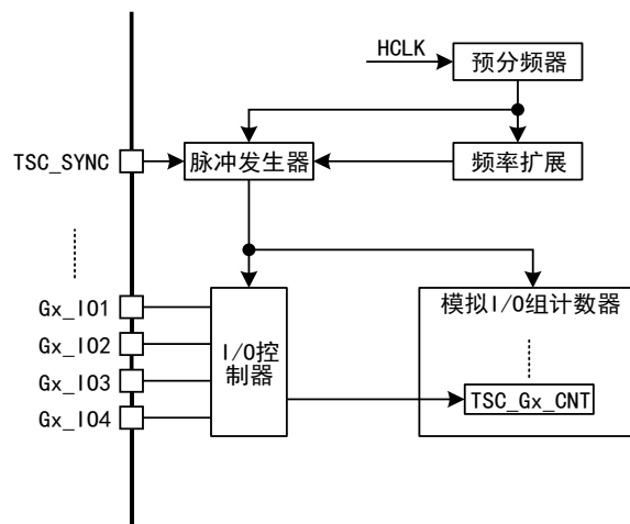
图 129 结构框图
