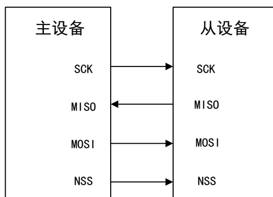
图 101 全双工模式连接
