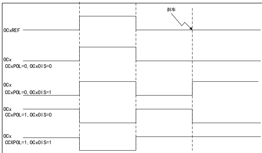
图 71 发生刹车事件的时序图
