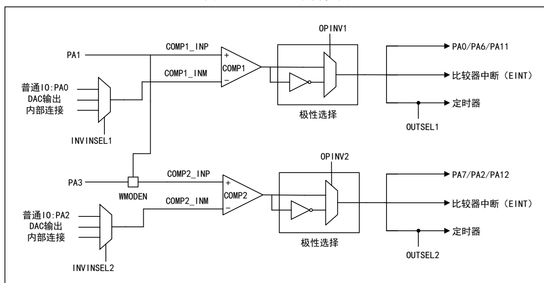
图 130 COMP 结构框图
