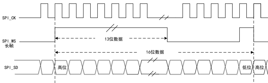
图 114 PCM 标准波形
