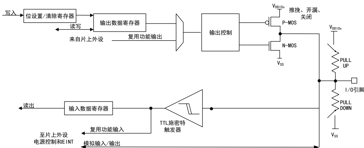
图 17 GPIO 结构框图
