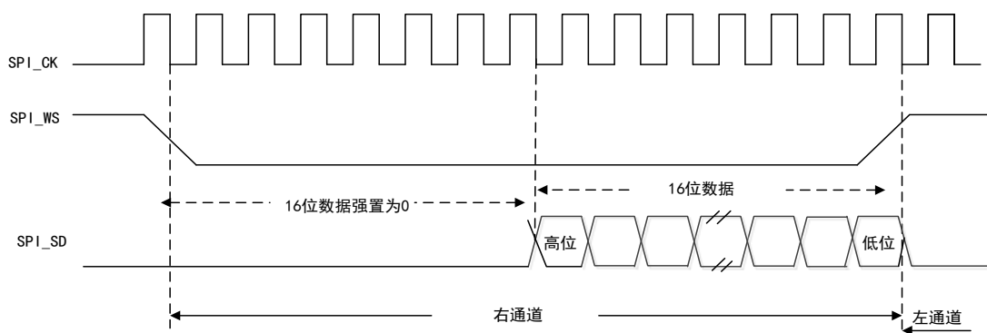
图 113 LSB 对齐标准下（16 位扩展至 32 位）
