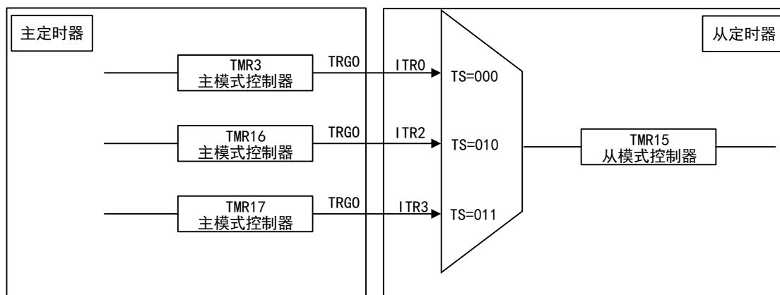
图 56 TMR15 与其它定时器互连
