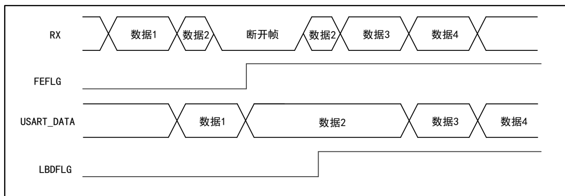
图 90 数据传输状态检测断开帧
