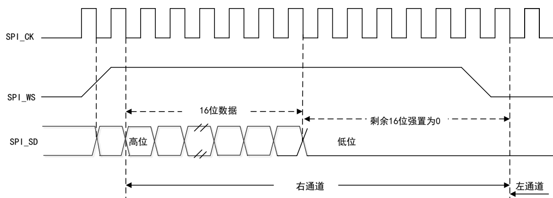
图 107 I2S 飞利浦协议波形（16 位扩展至 32 位）
