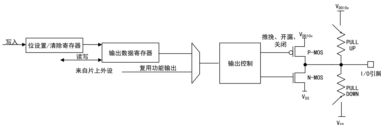
图 19 输出模式 I/O 结构
