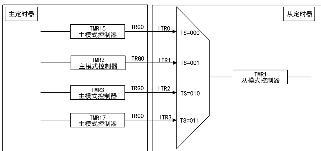
图 75 定时器 1 主/从模式的例子
