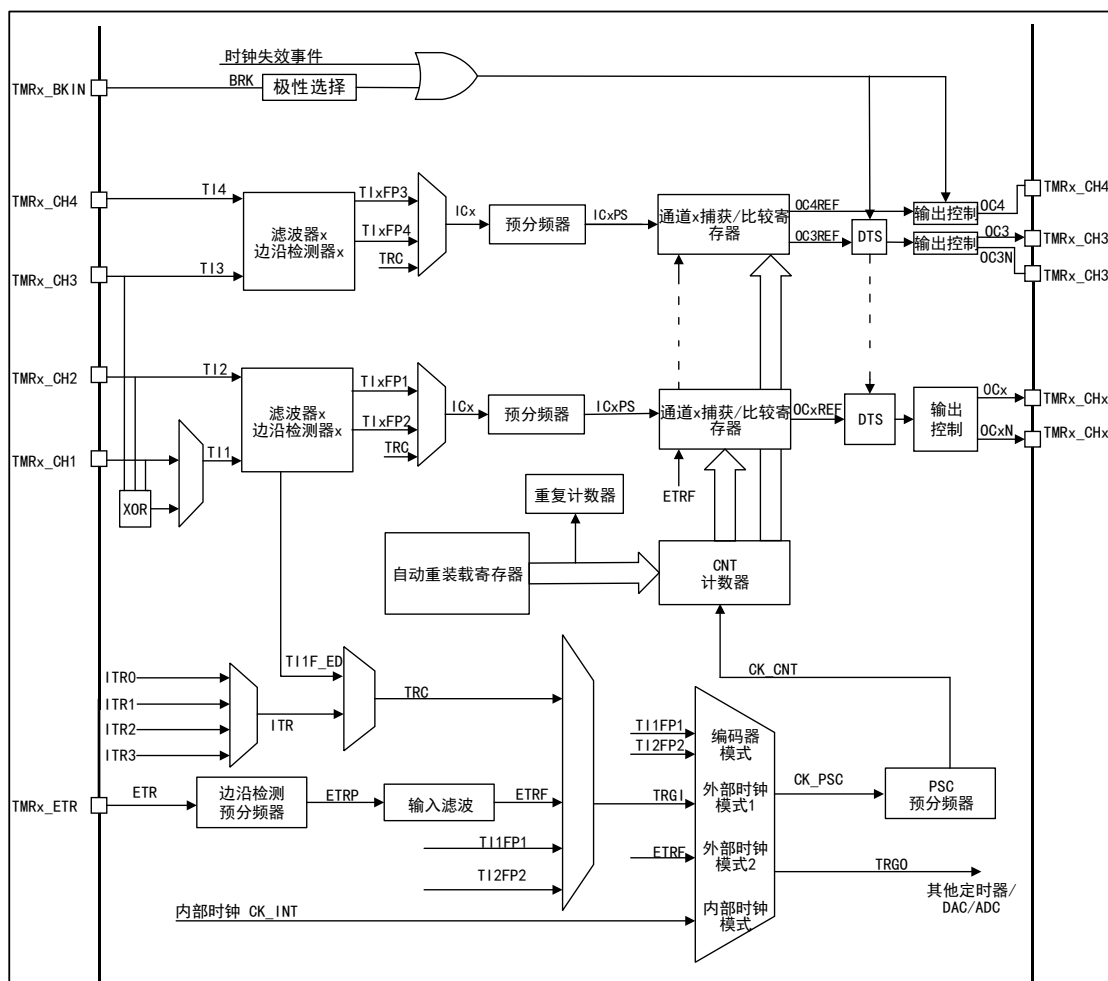
图 57 TMR1 结构框图
