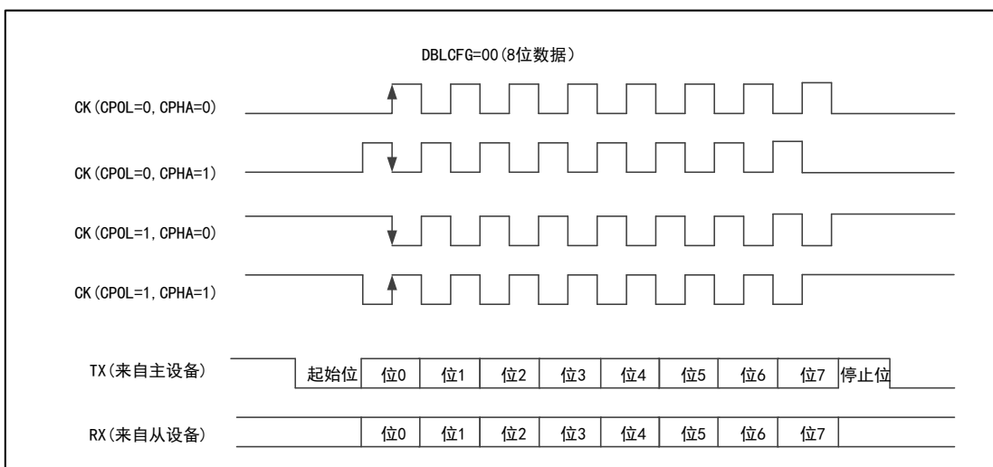
图 87 USART 同步传输时序图 (DBLCFG=00)
