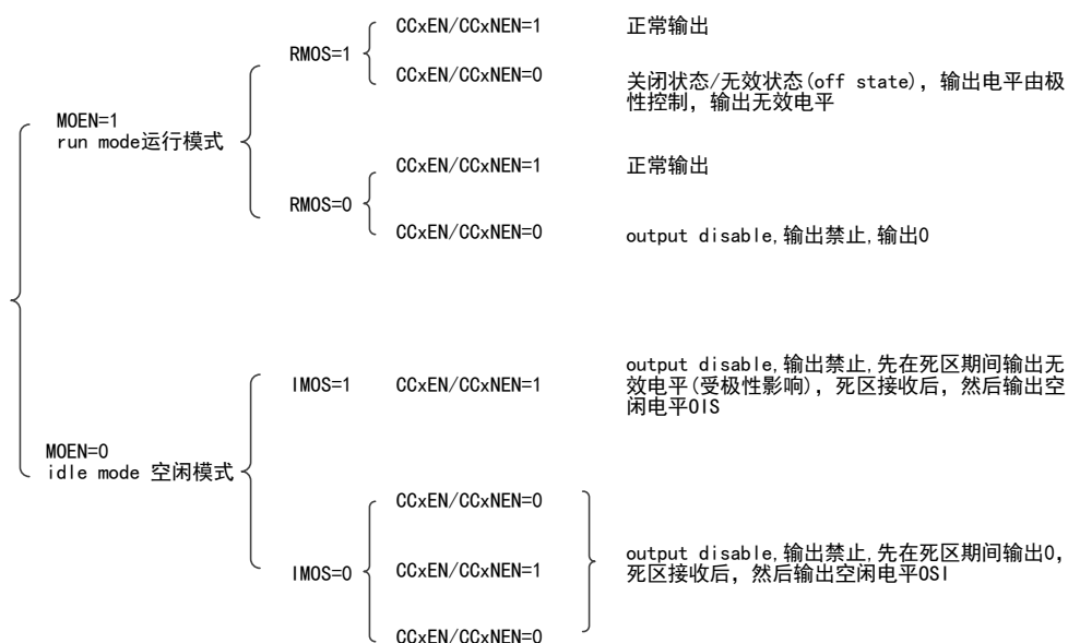
图 70 影响输出波形的寄存器结构关系
