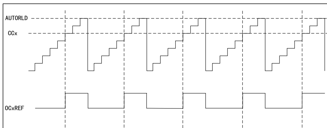
图 50 PWM2 向上计数模式的时序图
