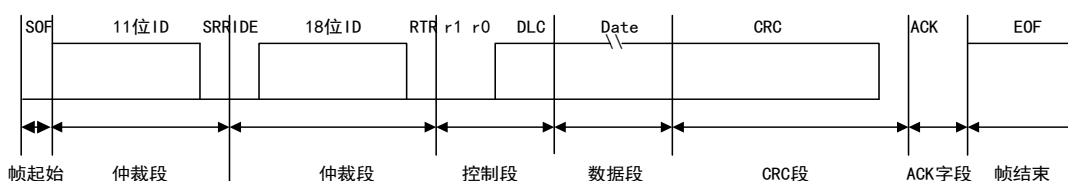
图 117 扩展数据帧
