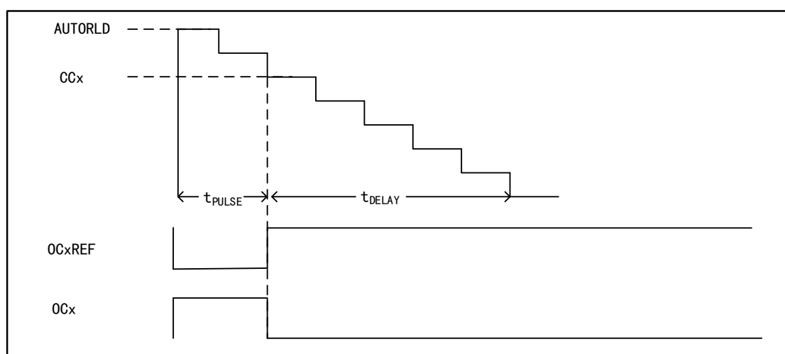
图 69 单脉冲模式下的时序图
