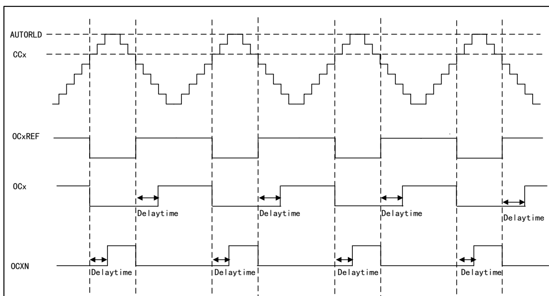
图 72 带死区插入的互补输出
