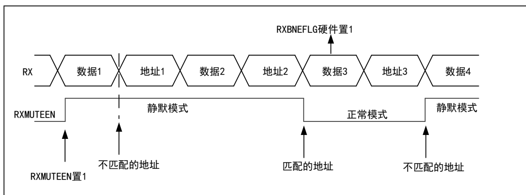
图 84 地址标记退出静默模式
