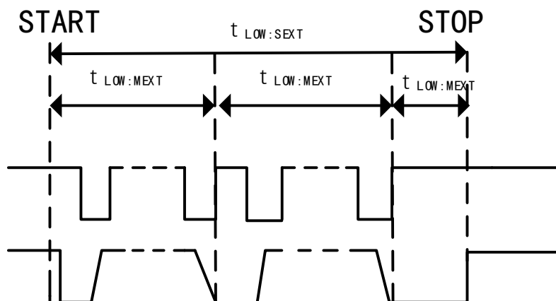
图 100 t_{LOW:SEXT} 与 t_{LOW:MEXT} 时间
