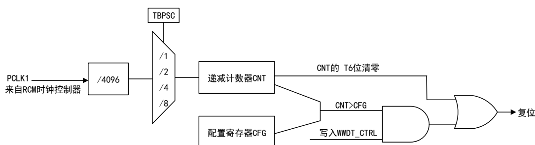
图 80 窗口看门狗功能框图
